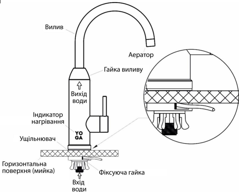
Рис. 2. Встановлення з виведенням кабелю живлення під мийкою
