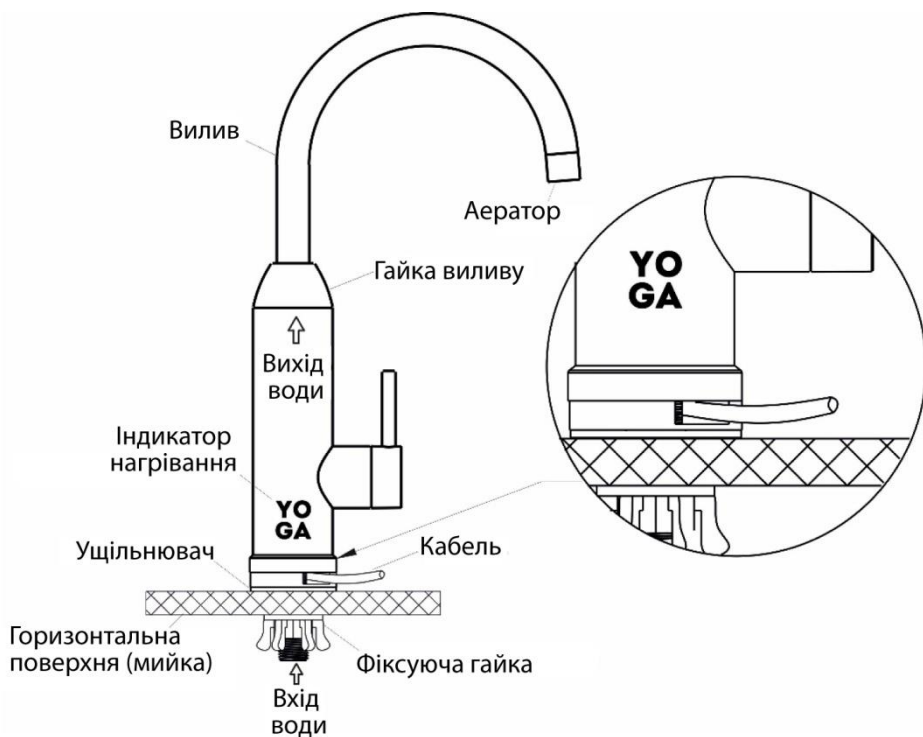
Рис. 1. Встановлення з виведенням кабелю живлення над мийкою
