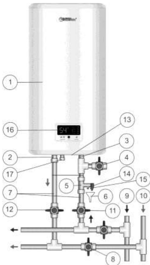
Рисунок 1. Схема підключення ЕВН до водопроводу
